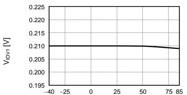
8. V_{IOV1} - T_a
