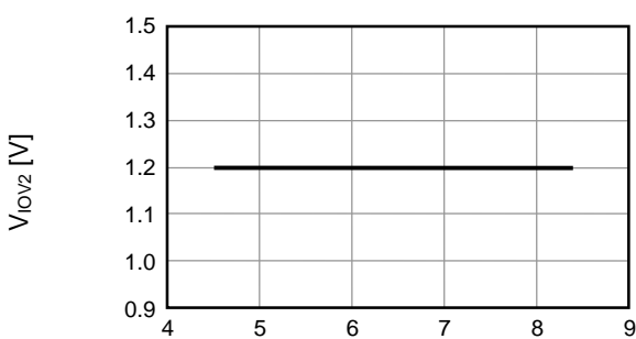
9. V_{IOV2} - V_{DD}
