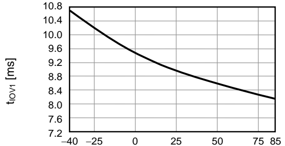
12. t_{IOV1} - T_a
