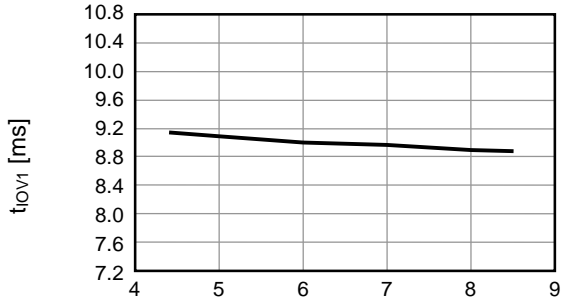
11. t_{IOV1} - V_{DD}
