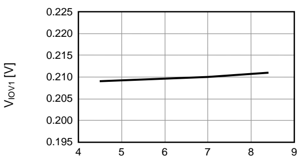
7. V_{IOV1} - V_{DD}
