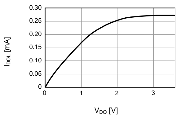
4. I_{DOL} - V_{DO}
