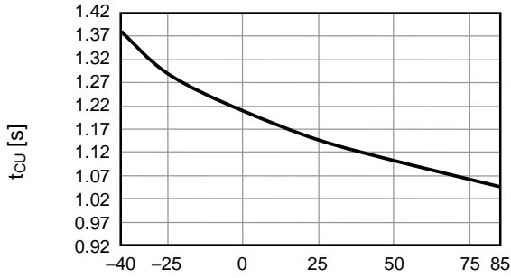
5. t_{CU} - T_a
